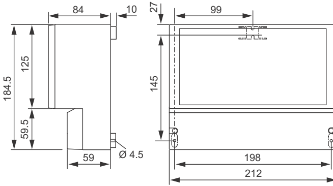
Abb. 3 Conex® DIA-G
