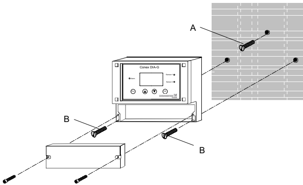
Abb. 6 Montagezeichnung
