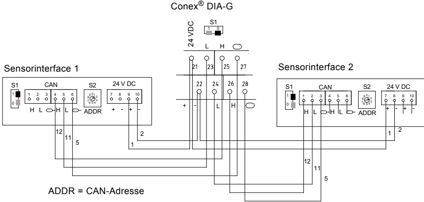
Abb. 13 Anschlussbeispiel 2
