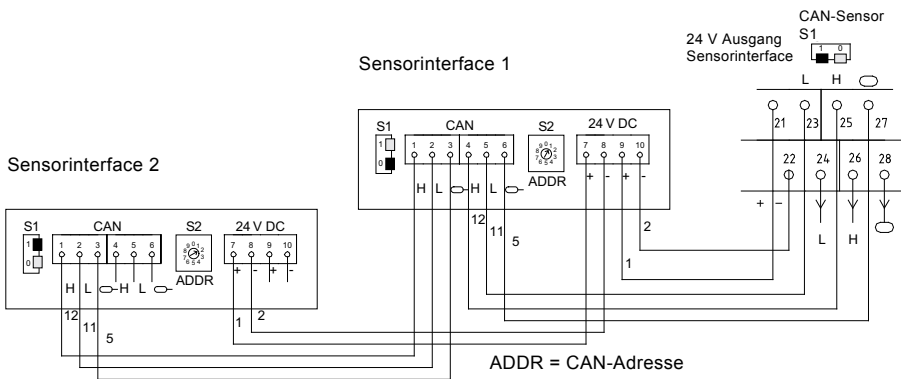
Abb. 12 Anschlussbeispiel 1
