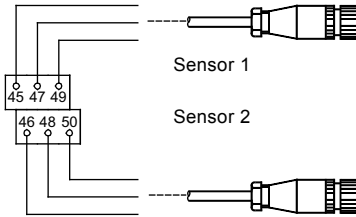
Abb. 11 Anschluss des amperometrischen Sensors
