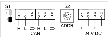
Abb. 10 Anschlussleiste des Sensorinterfaces Conex® DIA-G
