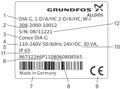
Abb. 1 Typenschild, Conex® DIA-G
