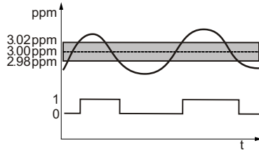
Abb. 15 Schalthysterese
