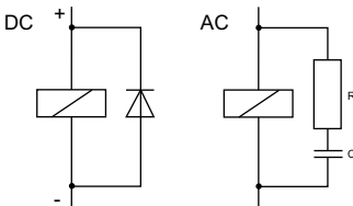
Abb. 9 Schutzschaltung, DC/AC
