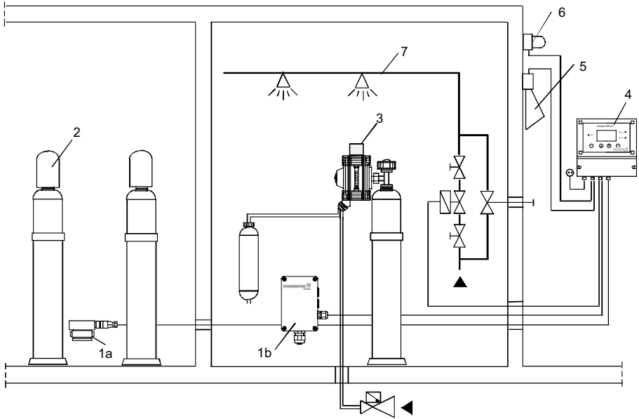
Abb. 2 Gaswarnsystem
