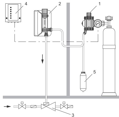
Abb. 12 Dosieranlage mit einer Chlorflasche
