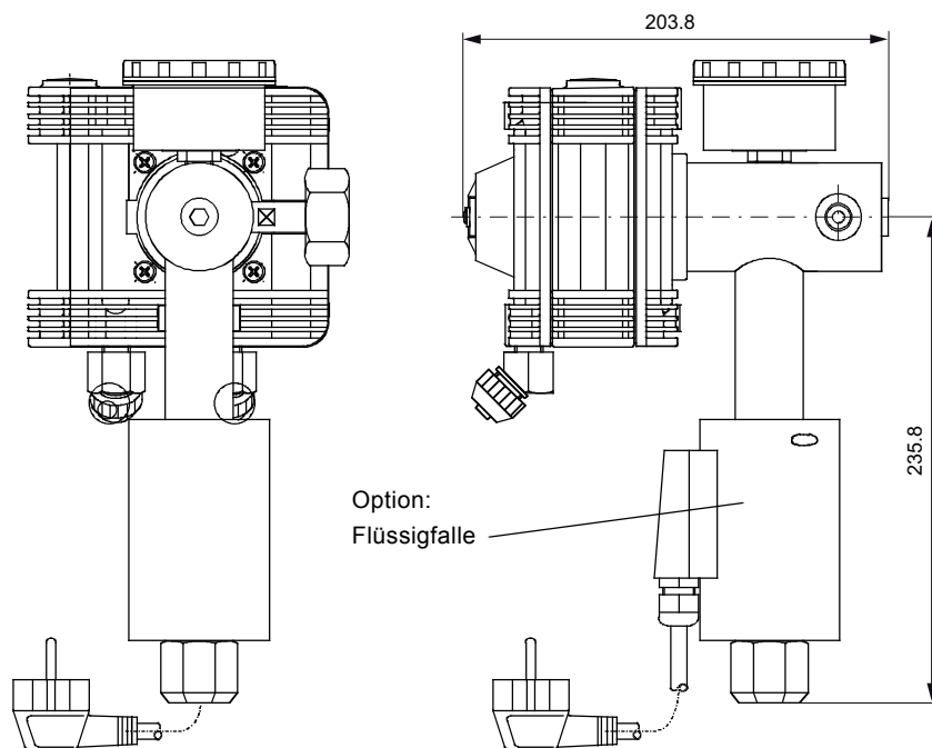
Abb. 6 Vakuumregler VGA-111 mit Flüssigfalle
