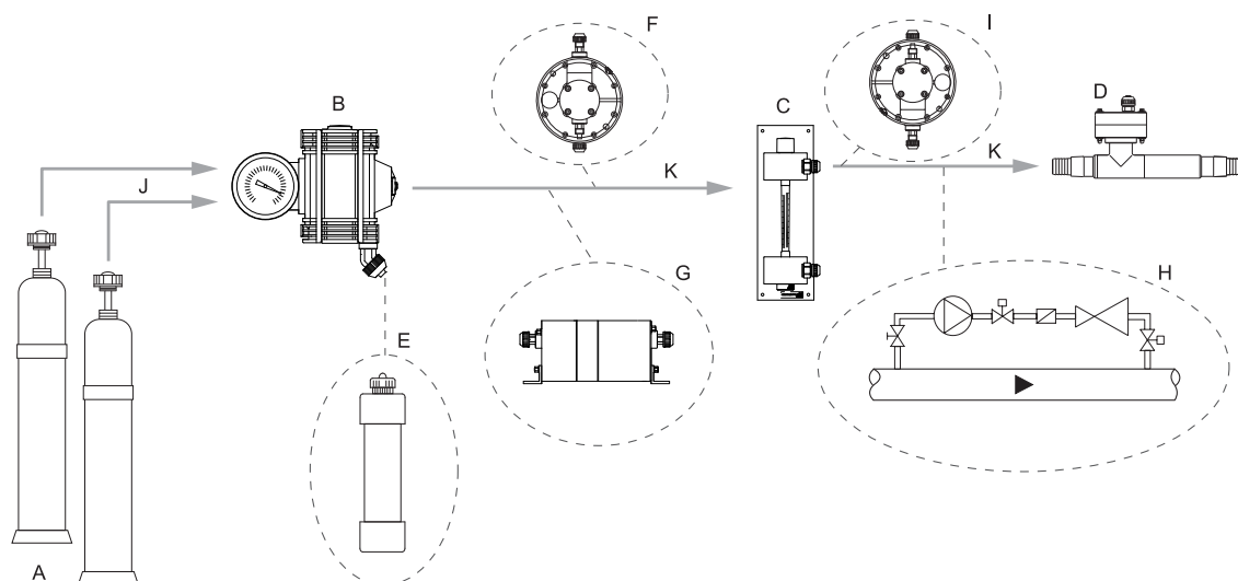
Abb. 10 Prinzip der Vakuum-Chlorgas-Dosieranlage
