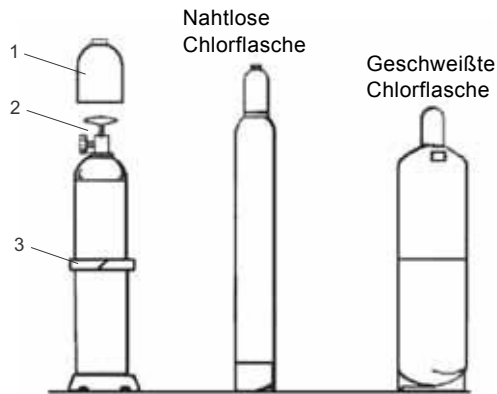
Abb. 1 Aufbau Flasche
