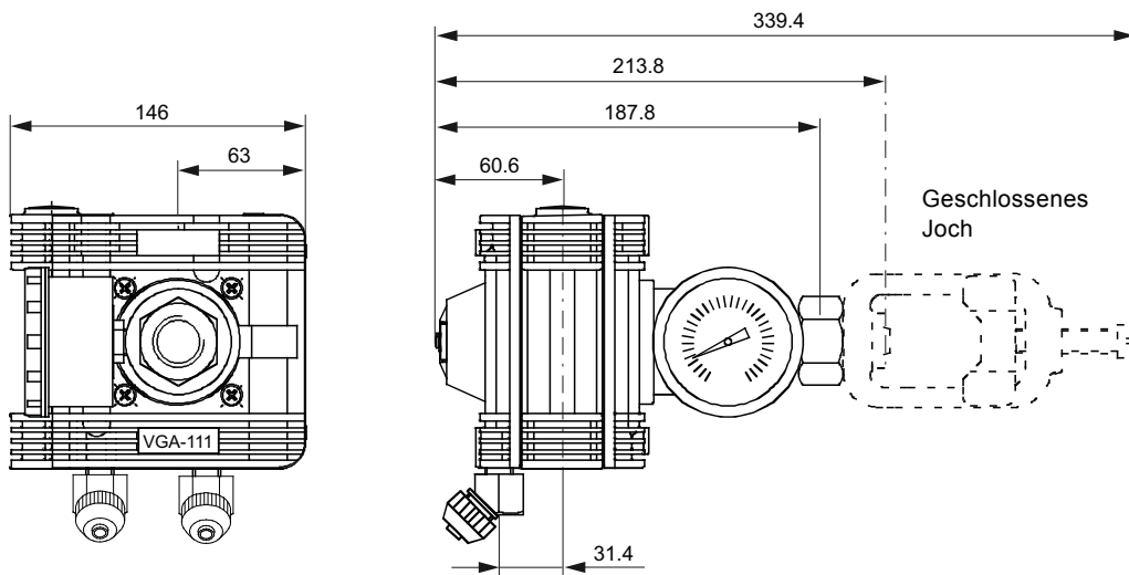
Abb. 5 Vakuumregler VGA-111
