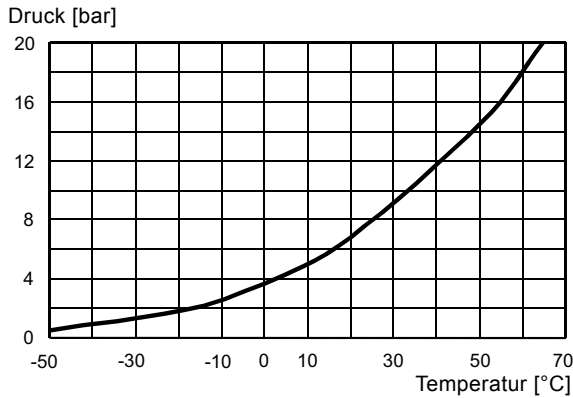
Abb. 7 Dampfdruckkurve von Chlor
