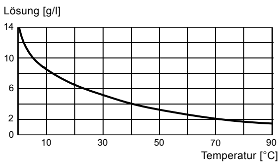
Abb. 8 Löslichkeit von Chlorgas in Wasser
